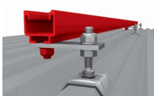
Illustration de la vis de fixation panneaux solaires, de l'adaptateur et d'un rail
